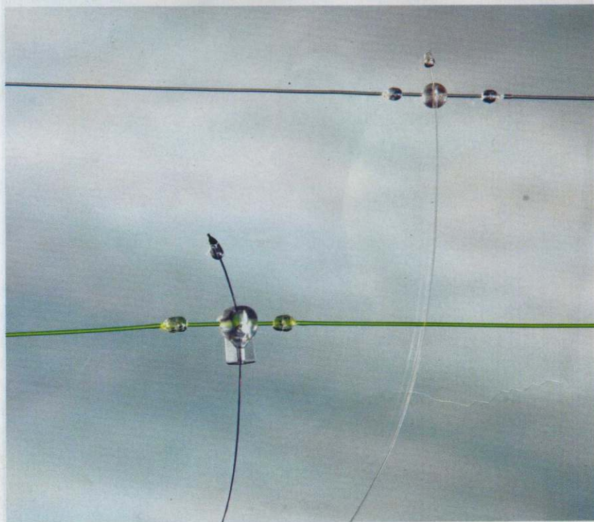
In basso a sinistra una Stonfo Beads Deep; in alto a destra una Clip Beads. Entrambe sono fermate con perline foro calibrato incollate
